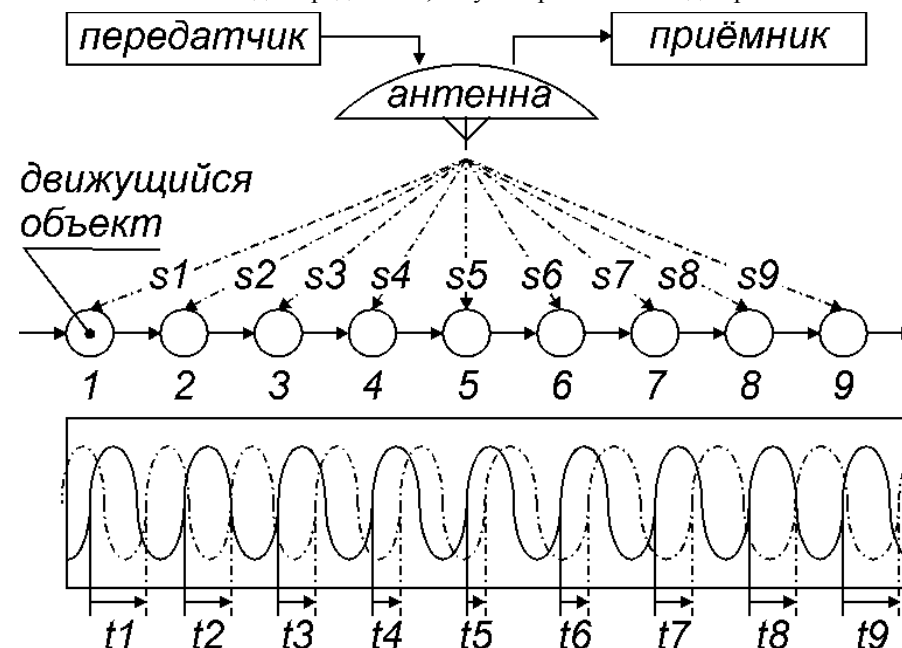
Рис. 3. Эффект Допплера.
