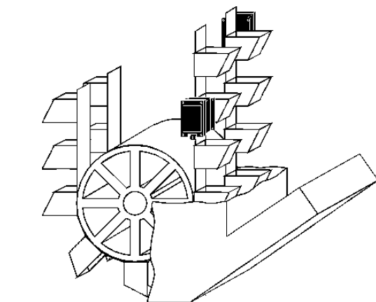
Рис. 7. Контроль скоростей лент двойной нории с металлическими ковшами.
